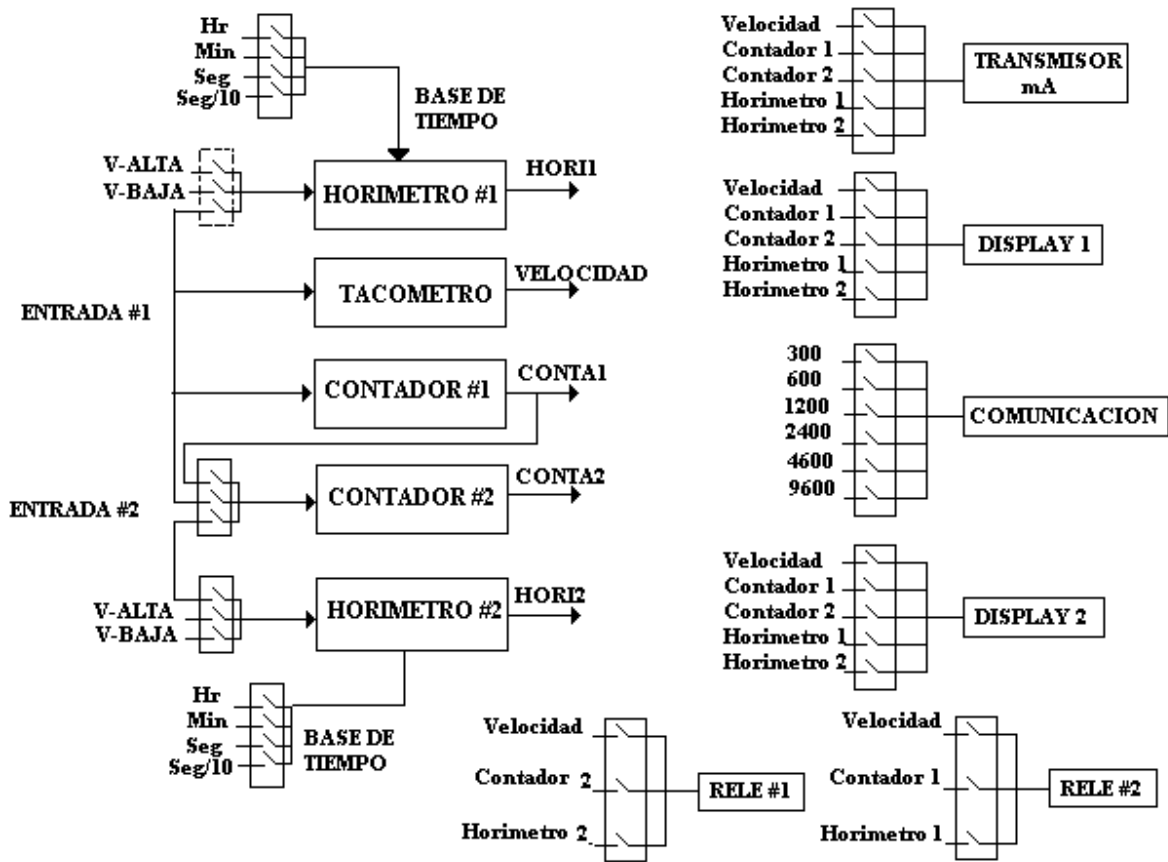
Fig. 4.1. ESTRUCTURA INTERNA DEL OMEGATROL 2530
